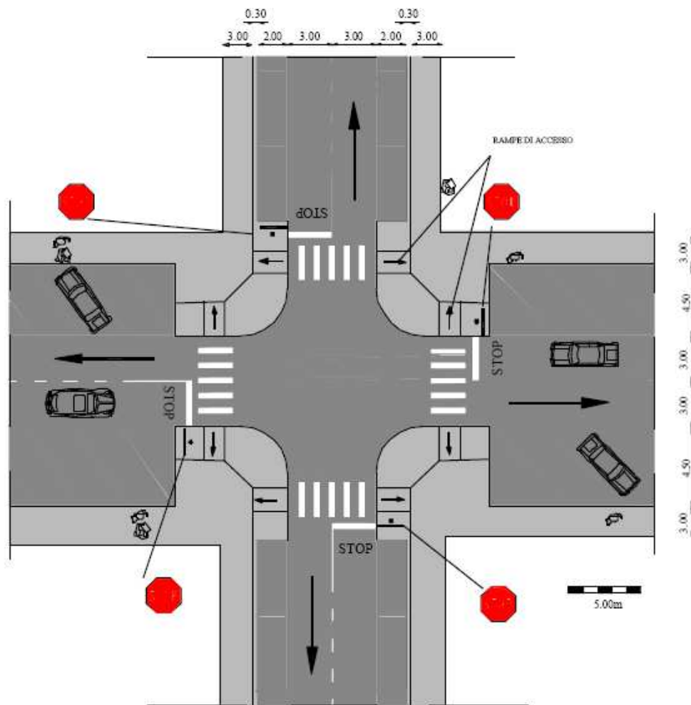
Figura 14 Allargamenti dei marciapiedi presso l'intersezione
