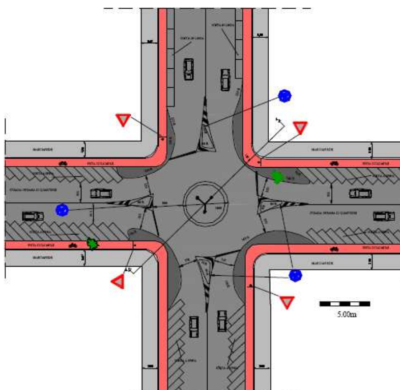
Figura 24 Esempi di minirotatoria con pista ciclabile
