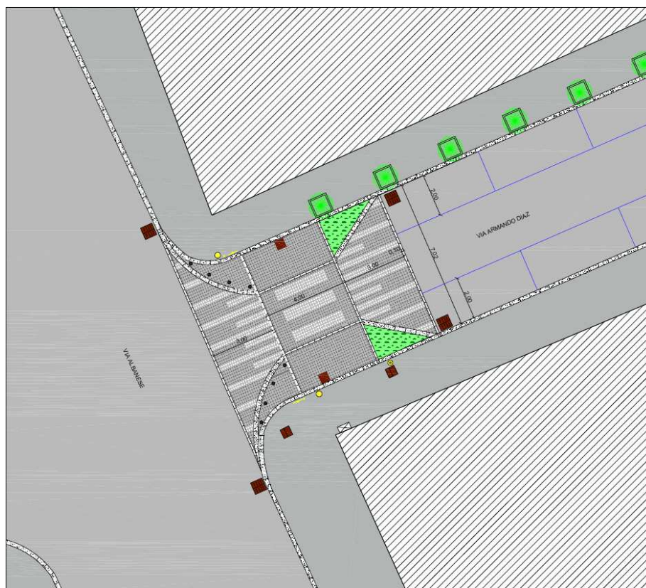
Figura 20 Esempio di porta per Zona a 30km/h e ZTPP
