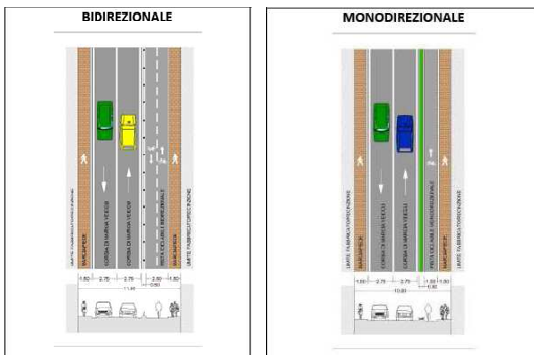
Figura 8 Esempi di pista ciclabile in sede propria in ambito urbano
