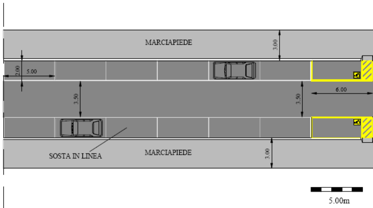
Figura 10 Le aree per la sosta su strada analizzata riguarda la sosta lungo il marciapiede o in linea.
