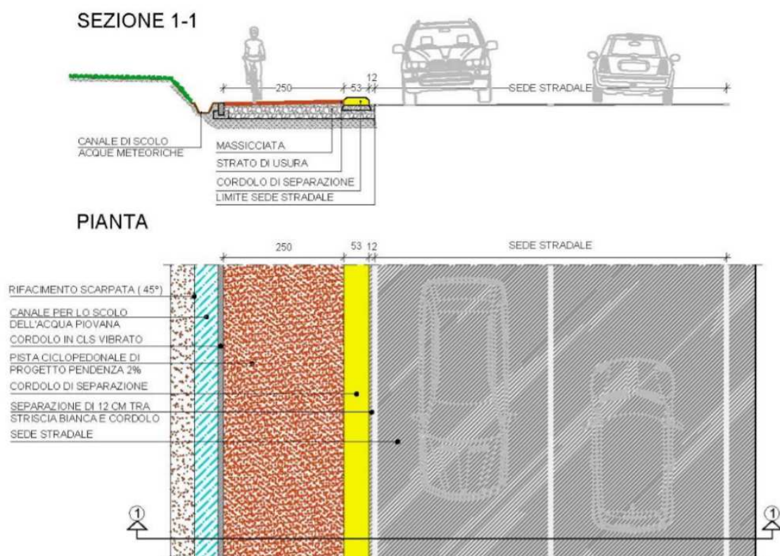
Figura 9 Esempio di pista ciclabile in sede propria su strada extraurbana secondaria
