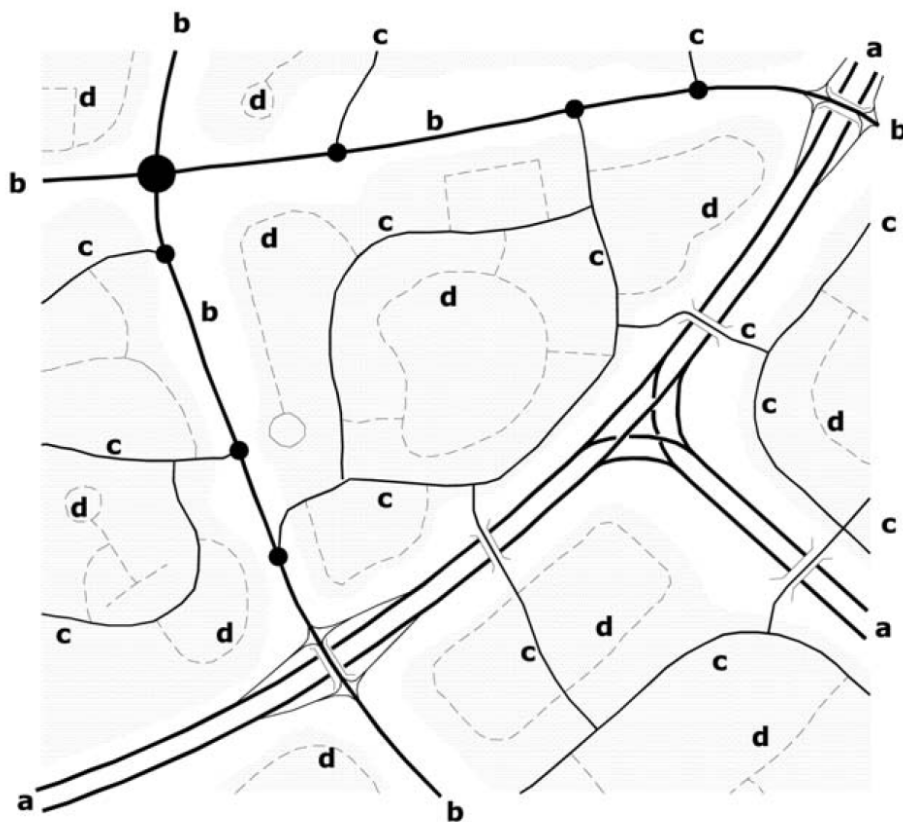
Figura 1 Caratteristiche gerarchiche e connessioni funzionali dei tipi di strade urbane
