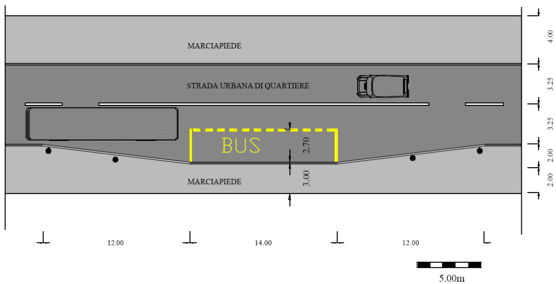
Figura 3 Tipo di fermata con piazzola di sosta
