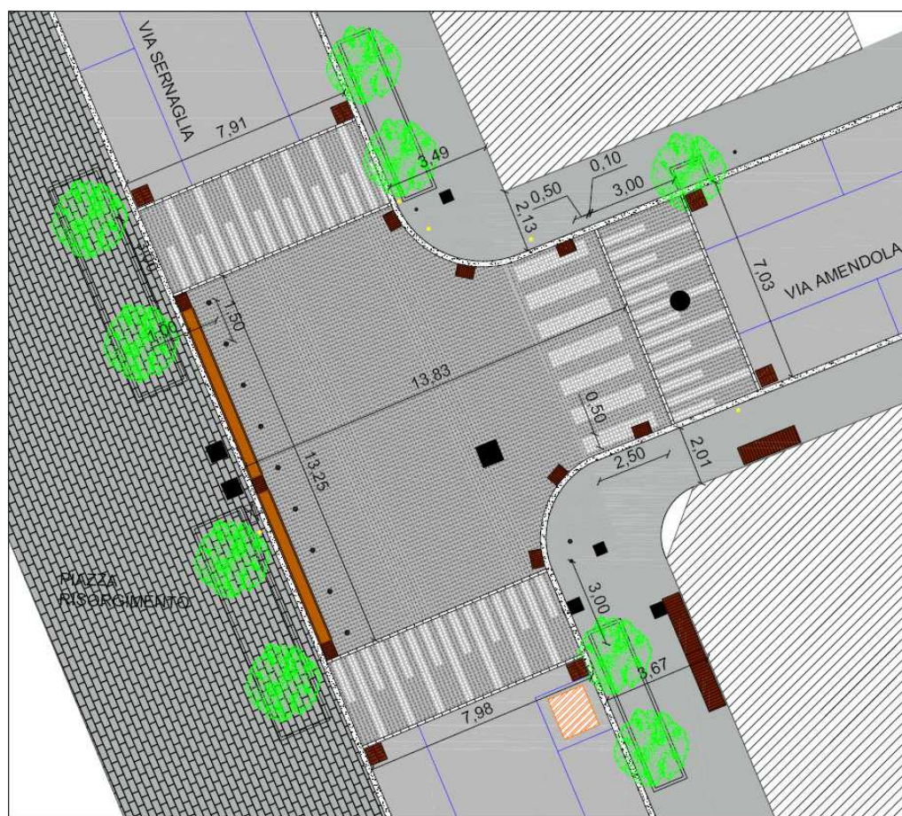
Figura 17 Esempio di Intersezione rialzata
