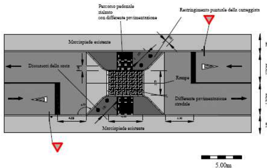
Figura 21 Esempio di “Restringimento puntuale della carreggiata con attraversamento pedonale rialzato”
