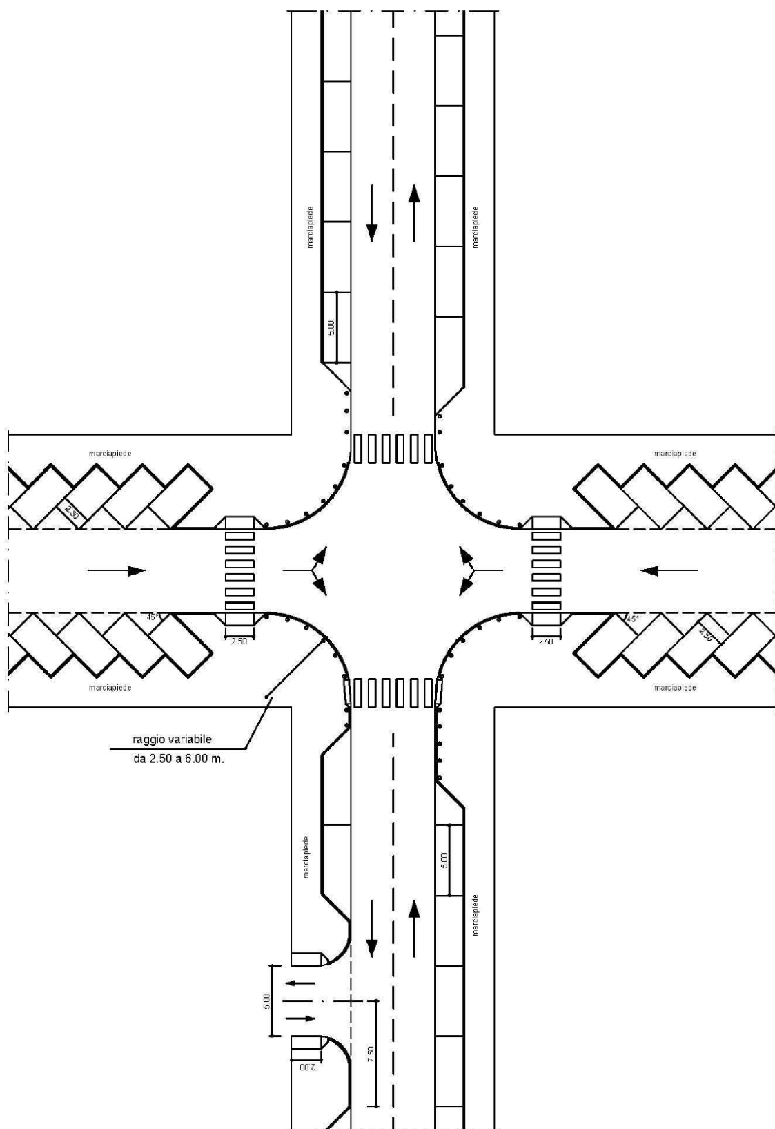
Figura 15 Organizzazione della sosta presso un'intersezione con strade a senso unico
