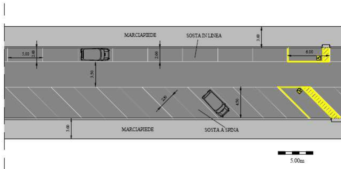
Figura 11 Le aree per la sosta su strada con stalli 45^\circ (a spina) e con stalli paralleli al marciapiede (in linea).
