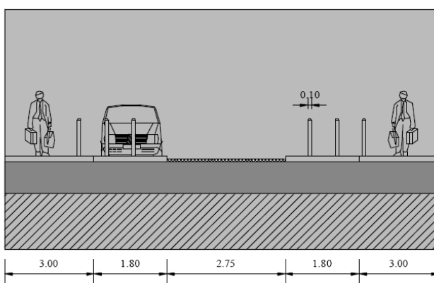
SEZIONE A-A
