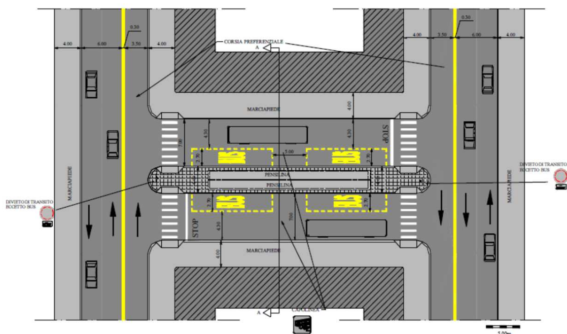
Figura 5 Esempio di capolinea di autobus di linea
