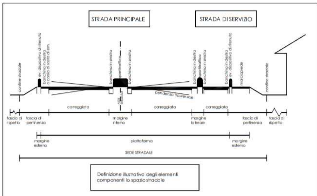
Figura 13 Elementi componenti lo spazio stradale
