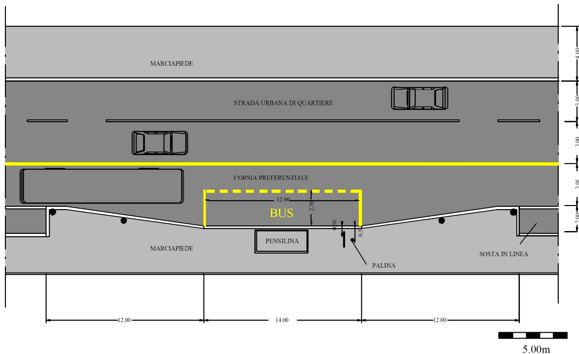
Figura 4 Tipo di fermata con piazzola di sosta con corsia preferenziale
