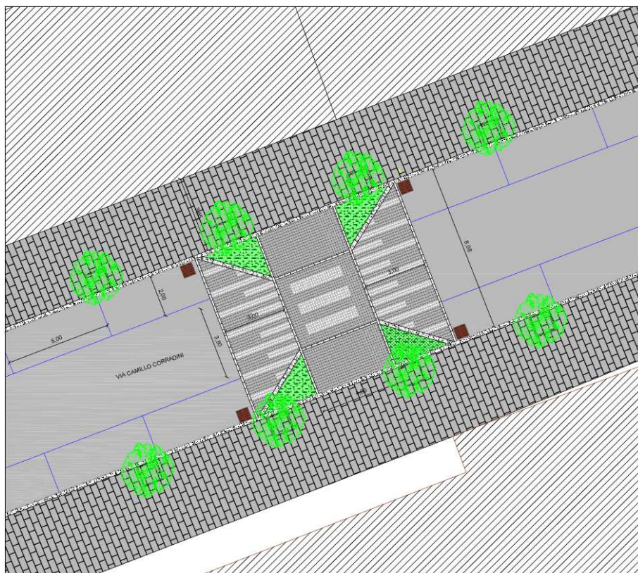
Figura 18 Esempio di attraversamento pedonale rialzato
