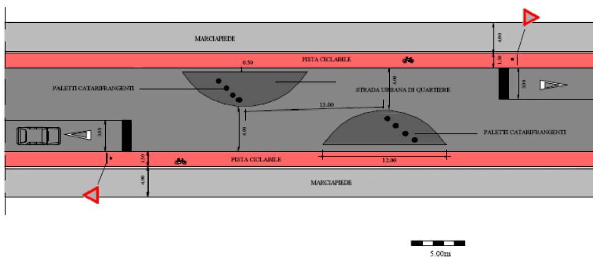
Figura 23 Esempio di Chicane con pista ciclabile
