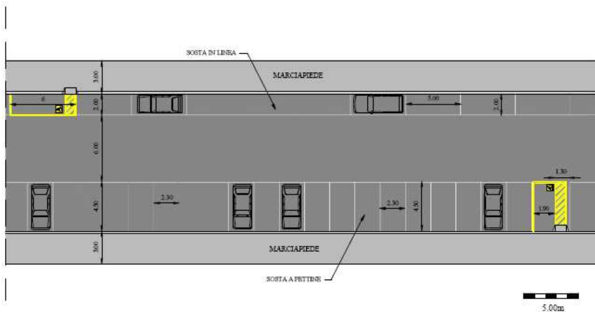
Figura 12 Le aree per la sosta su strada con stalli a 90° (a pettine) e con stalli paralleli al marciapiede (in linea).
