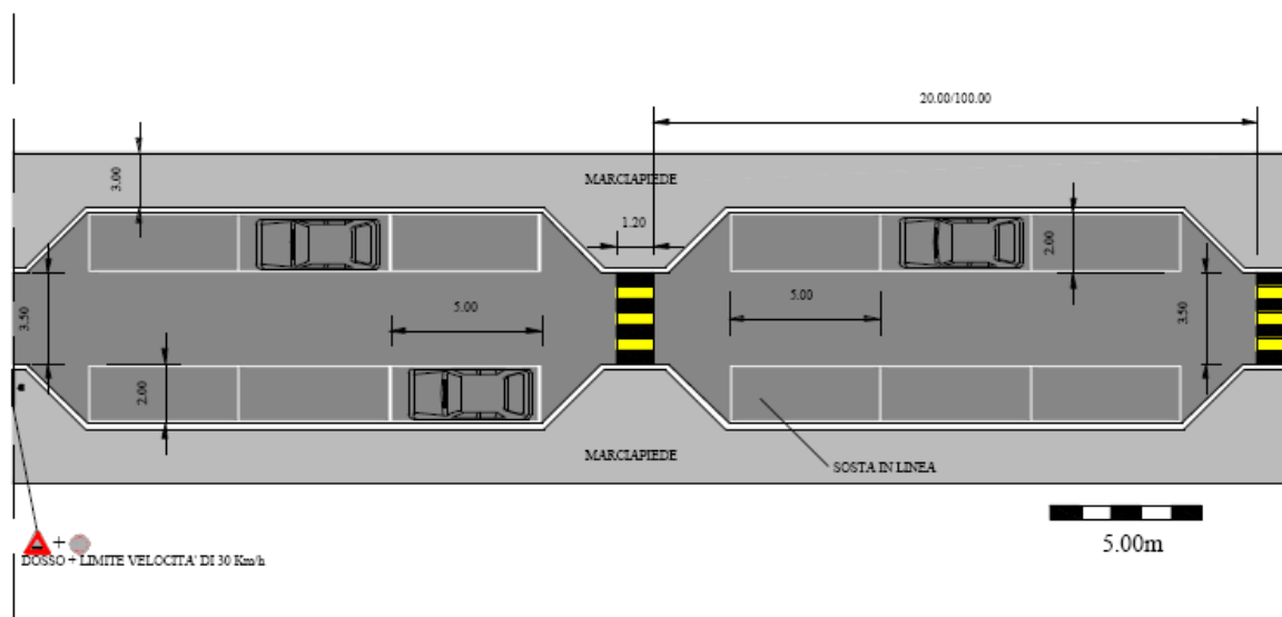
Figura 18 Esempio di attraversamento pedonale rialzato
