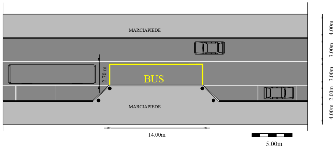
Figura 2 Fermata di autobus con avanzamento del marciapiede o bus stop boarder
